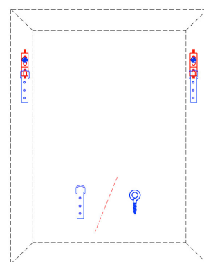
Accrochage par attaches ou pitons latéraux
